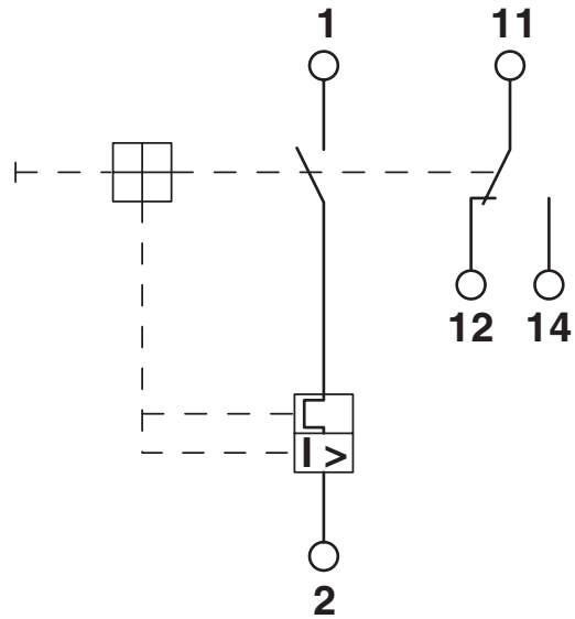
Koblingsskjema
