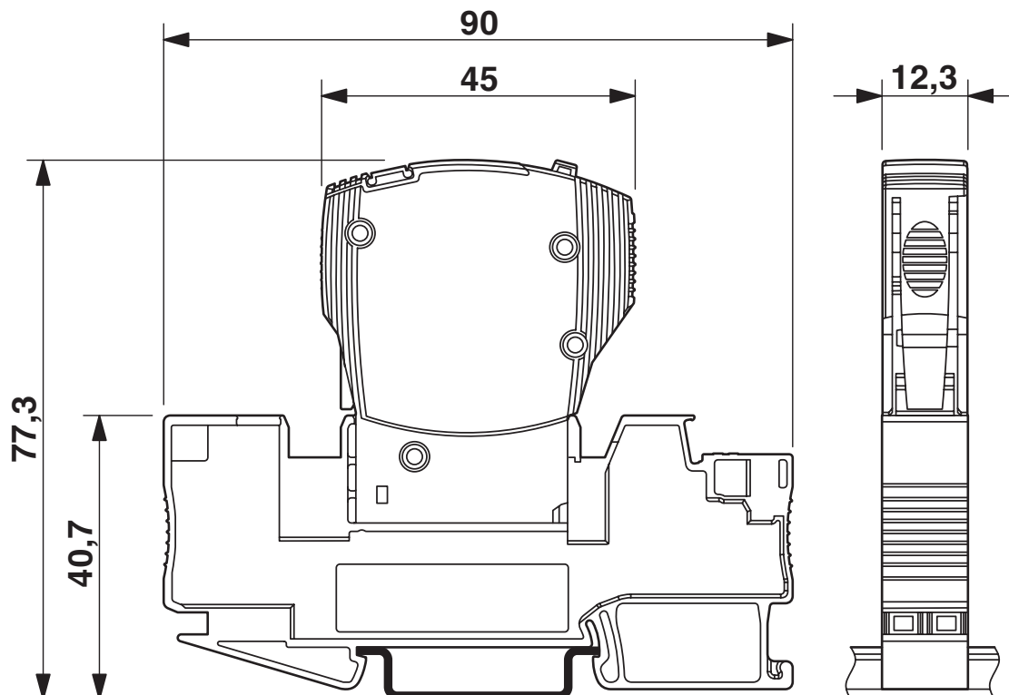
Målskisse
