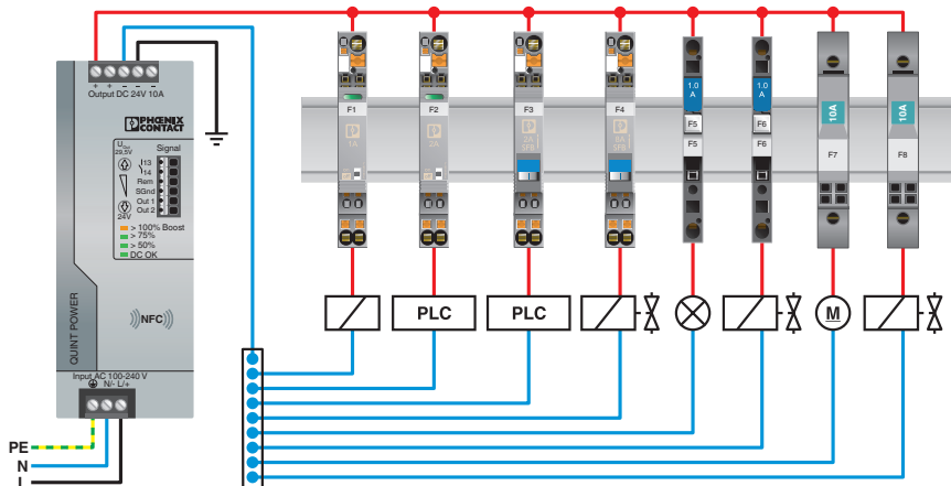
Applikasjonstegning
