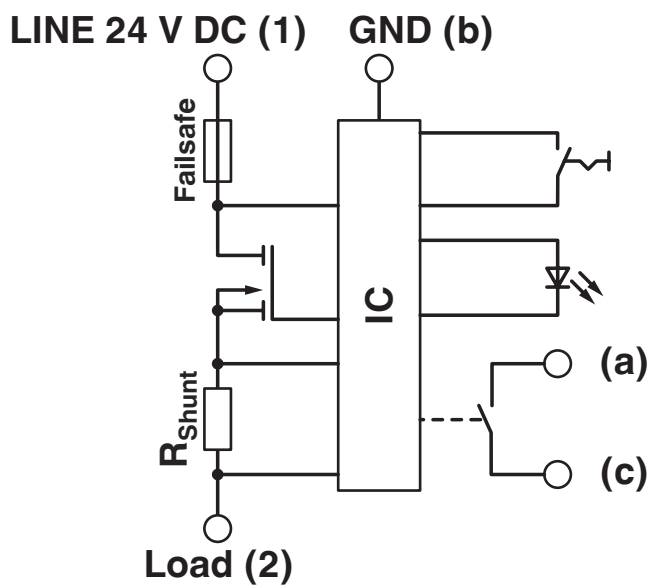
Koblingsskjema
