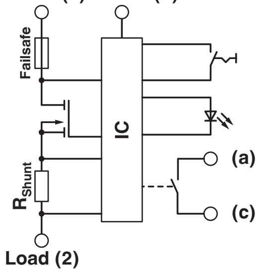
Koblingsskjema
