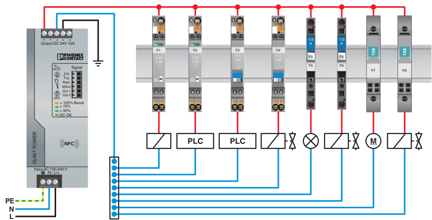
Applikasjonstegning
