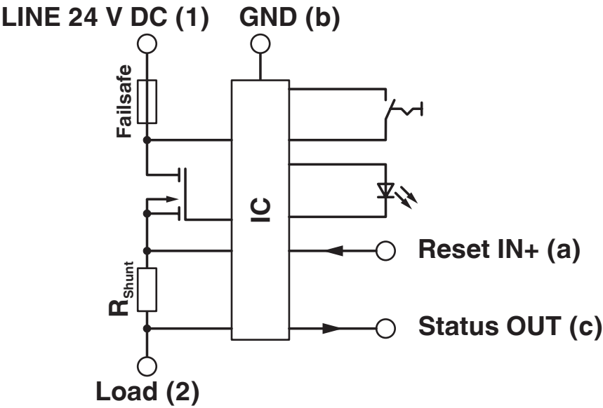
Koblingsskjema
