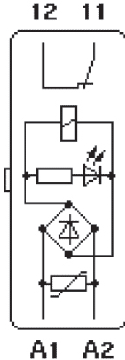
Koblingsskjema
