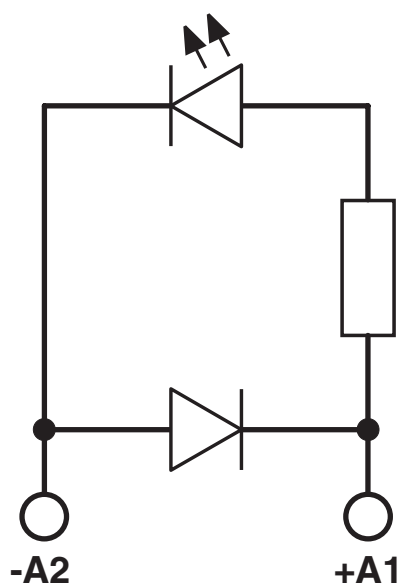
Koblingsskjema
