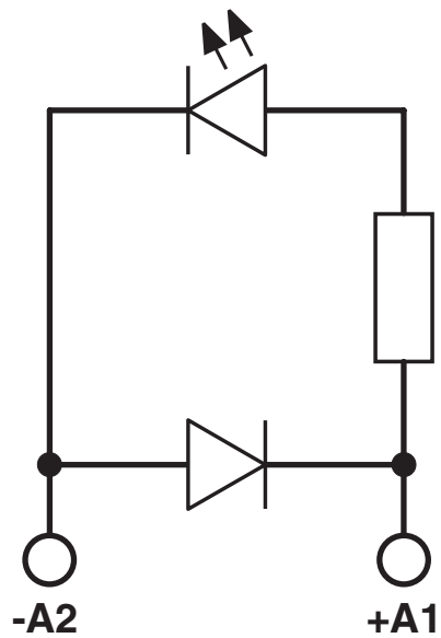
Koblingskjema
