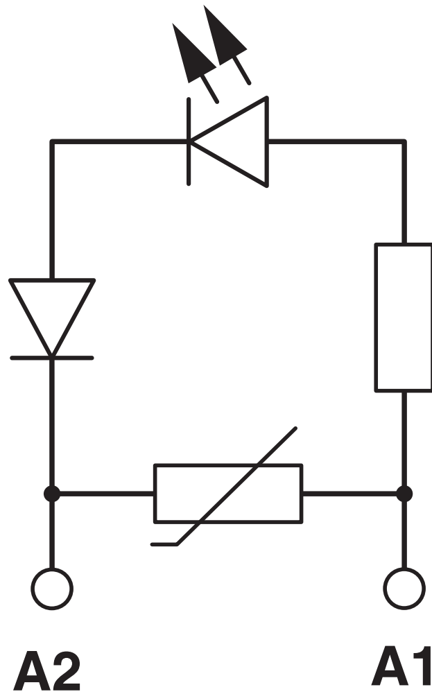
Koblingsskjema
