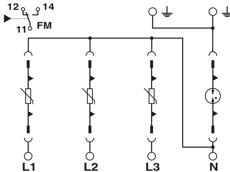
Koblingsskjema
