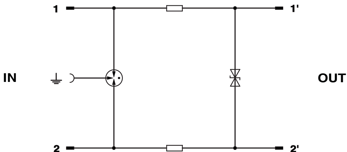
Koblingsskjema
