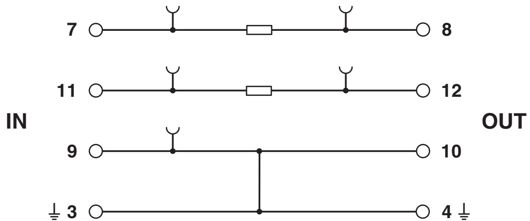
Koblingsskjema
