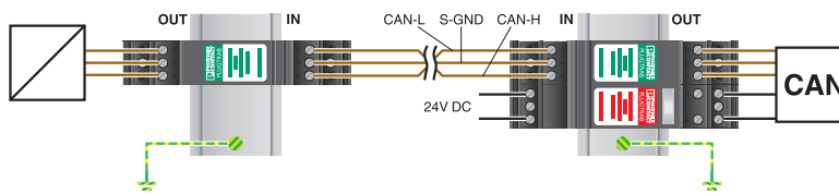
Applikasjonstegning
