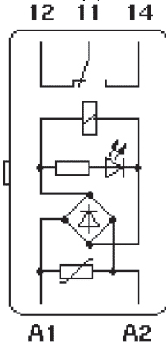
Koblingsskjema
