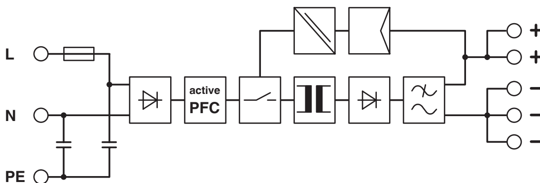
Blokkskjema
