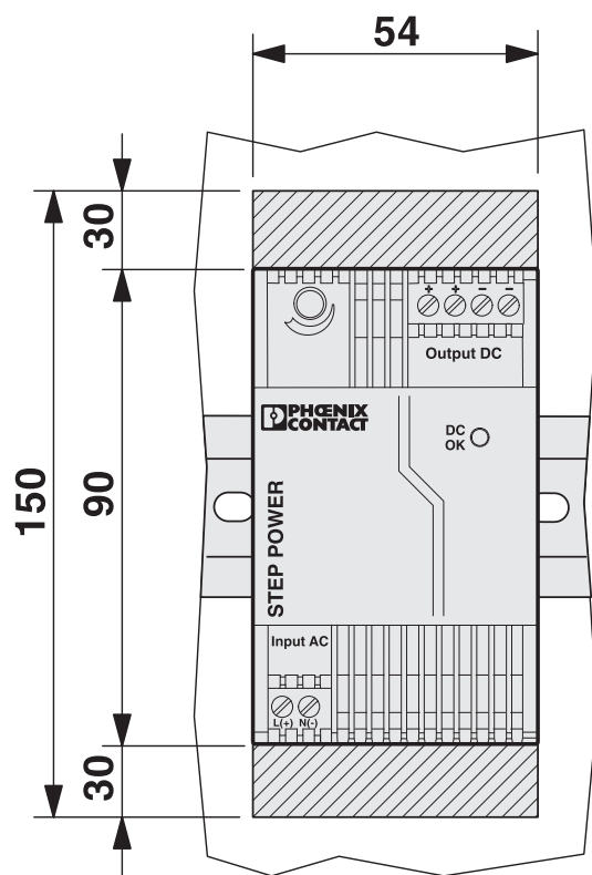
Målskisse
