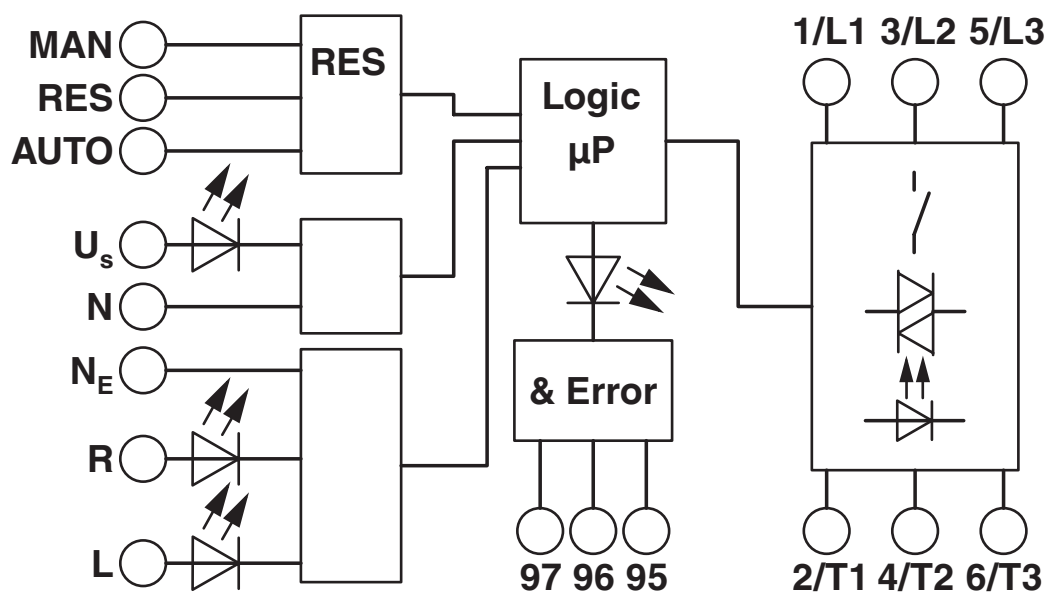
Blokkskjema
