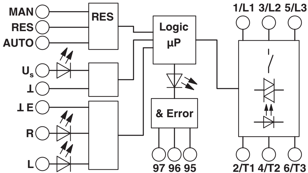
Blokkskjema
