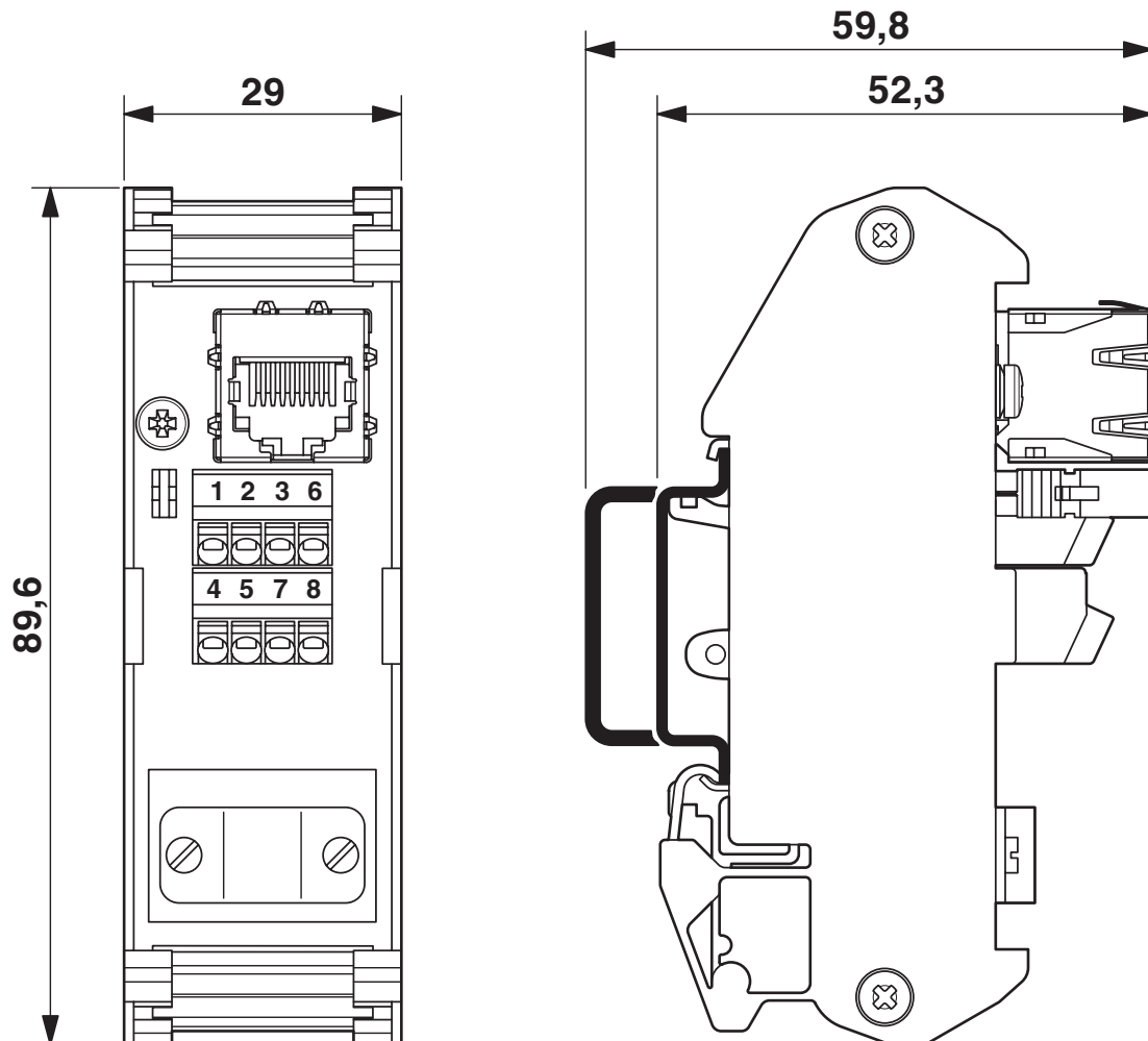
Målskisse
