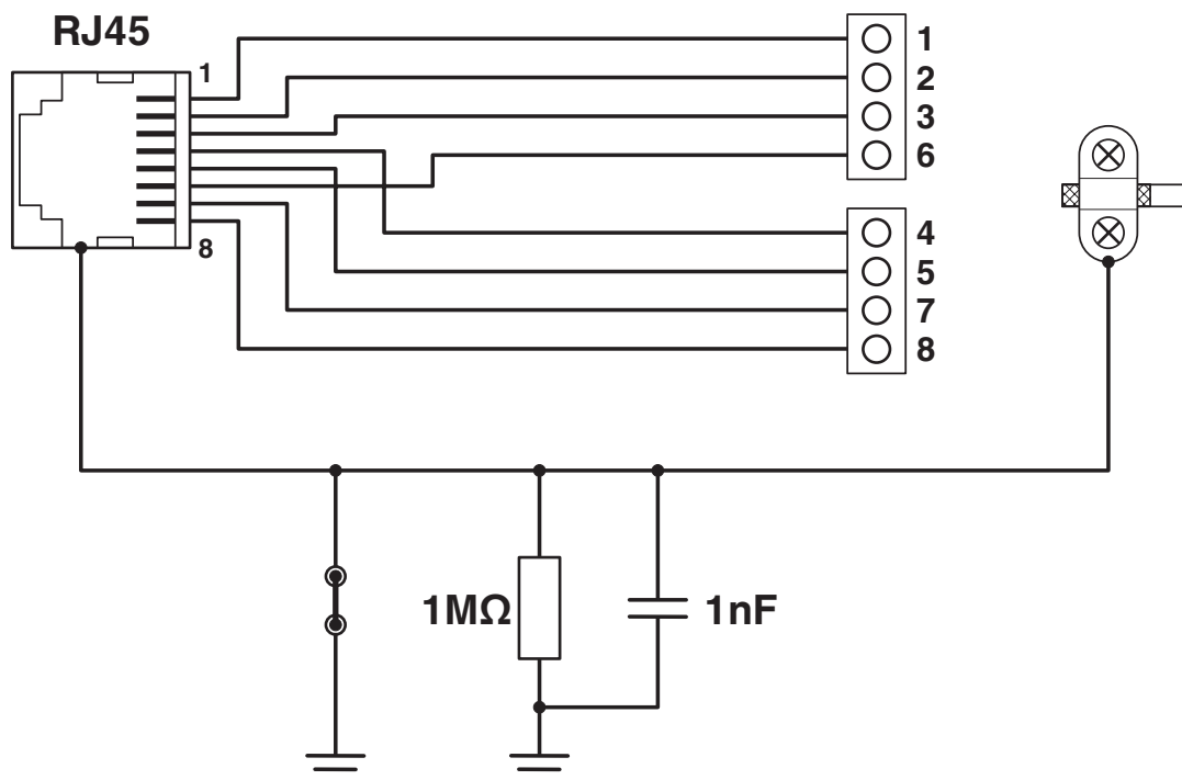
Koblingsskjema
