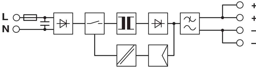
Blokkskjema
