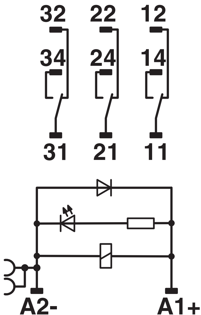
Koblingsskjema
