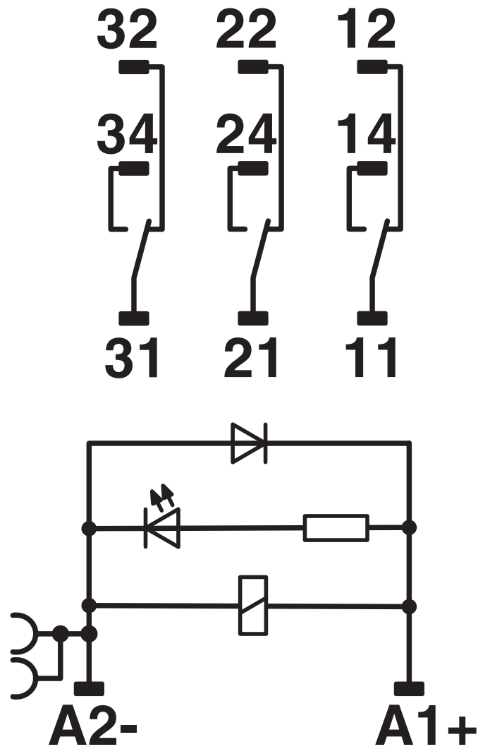
Koblingskjema
