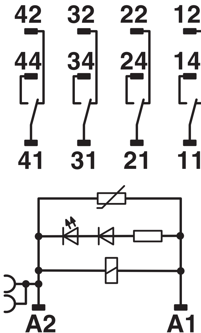
Koblingsskjema
