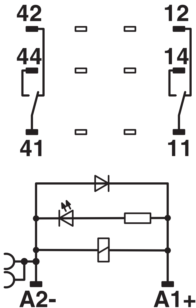
Koblingsskjema
