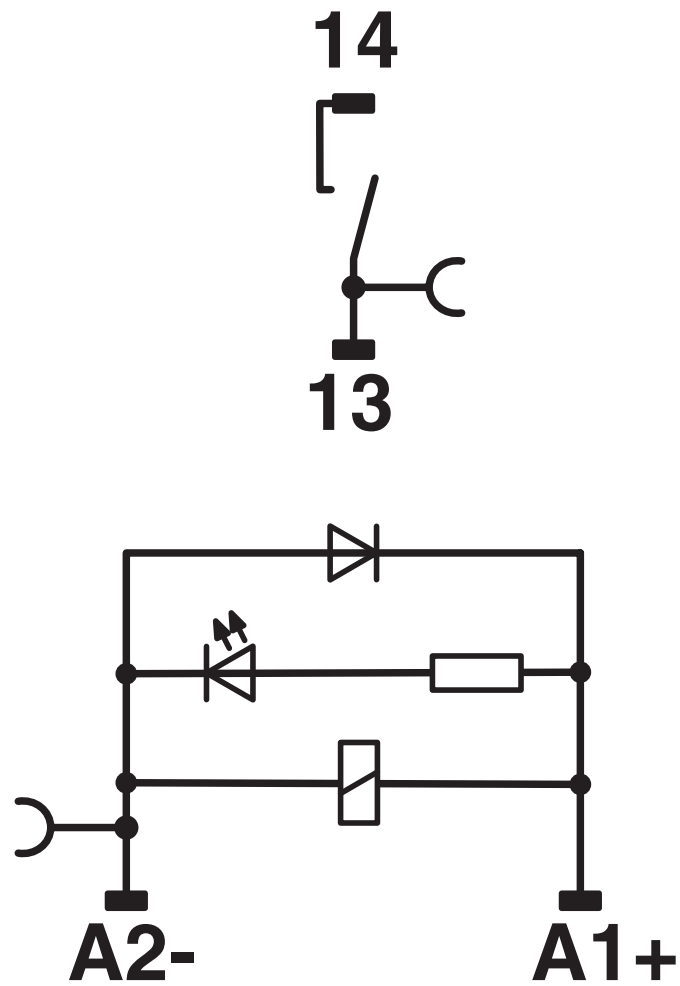
Koblingsskjema
