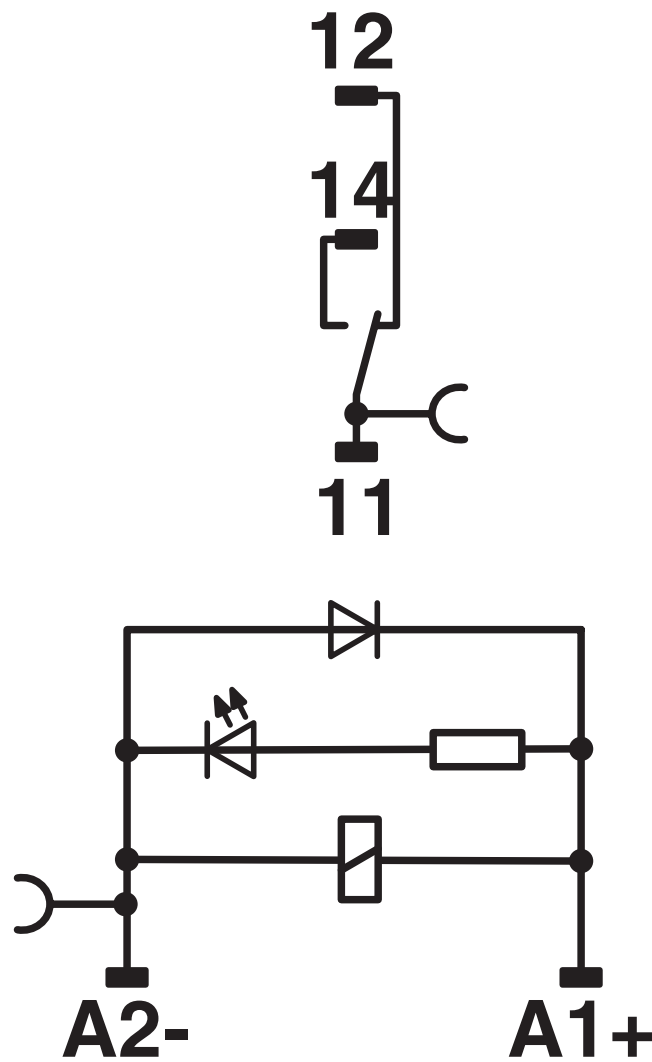
Koblingsskjema
