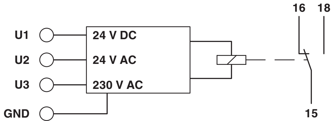
Blokkskjema
