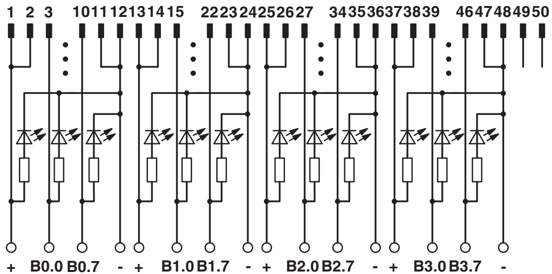
Koblingsskjema
