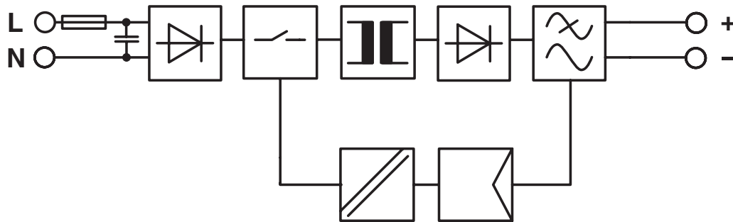
Blokkskjema
