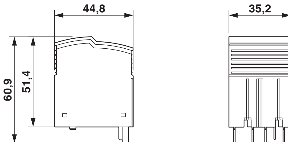
Målskisse
