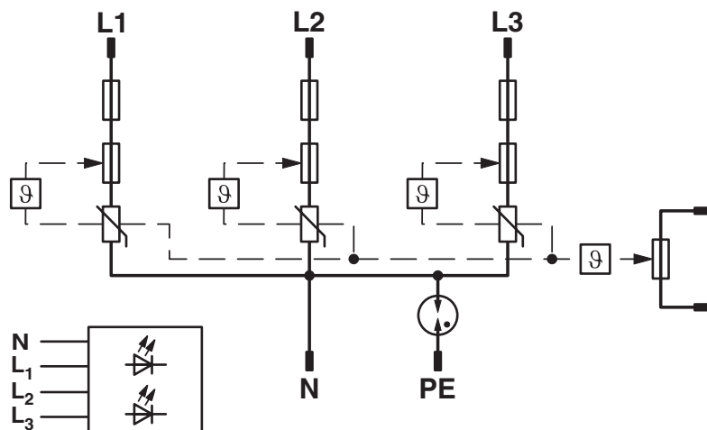
Koblingsskjema
