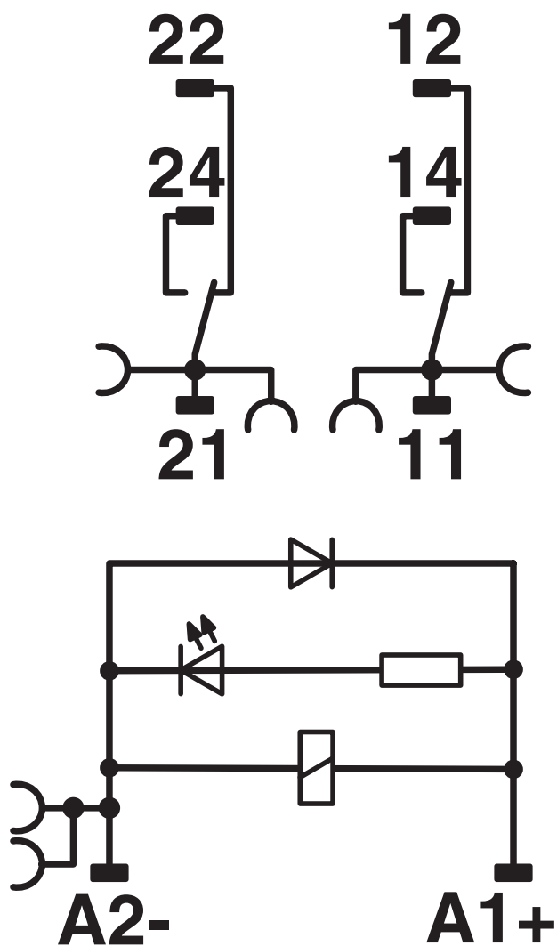
Koblingsskjema
