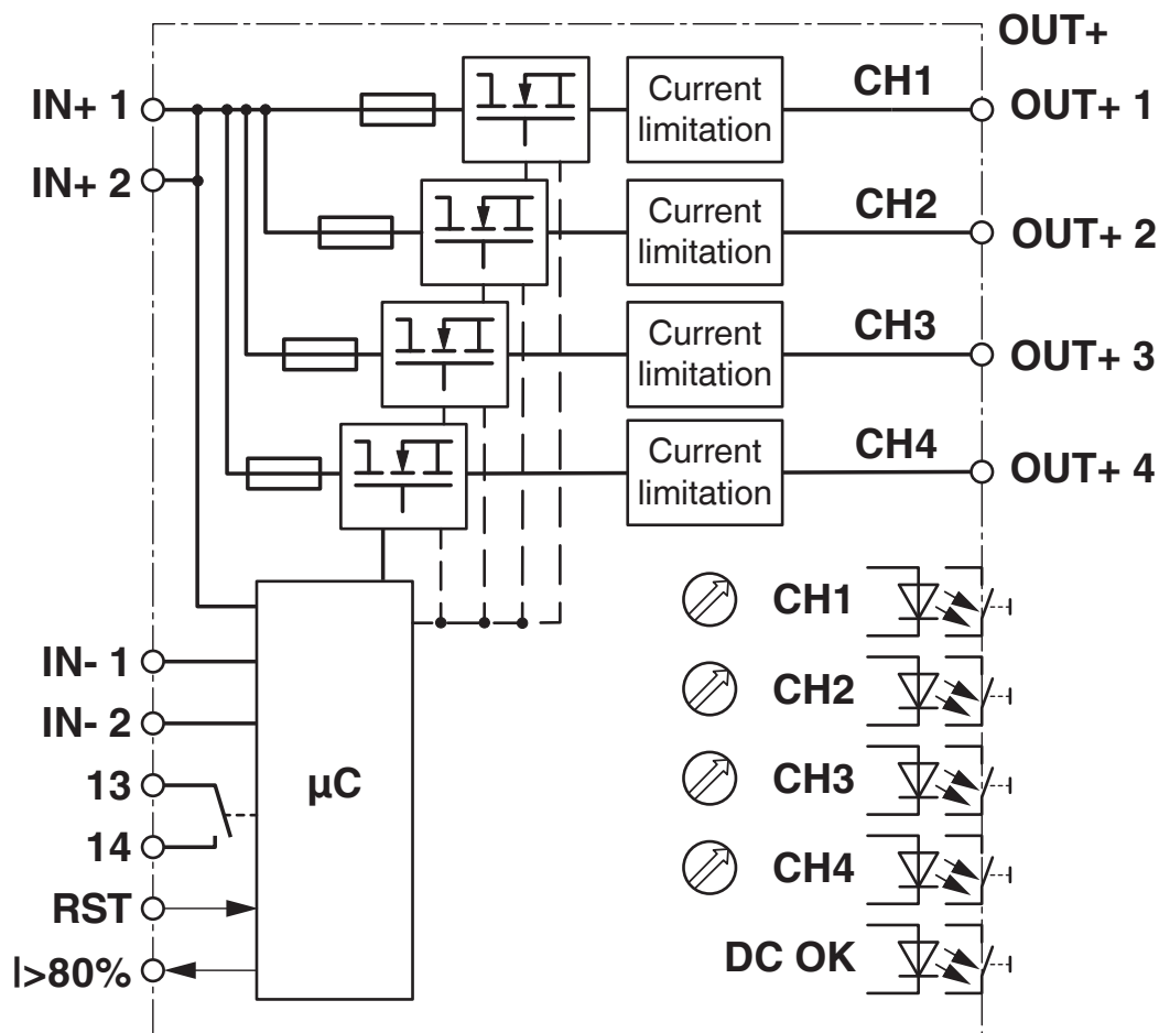
Blokkskjema
