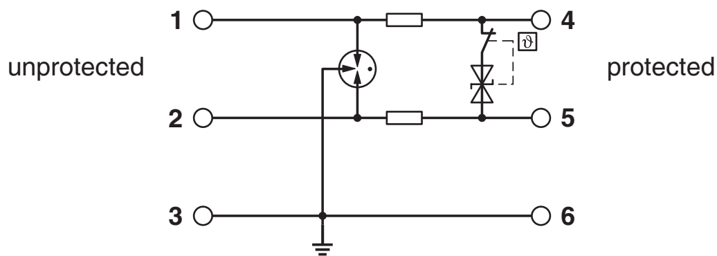
Koblingsskjema
