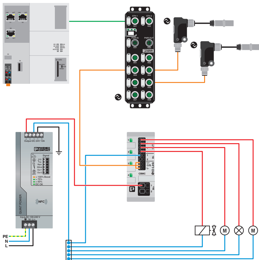
Applikasjonstegning
