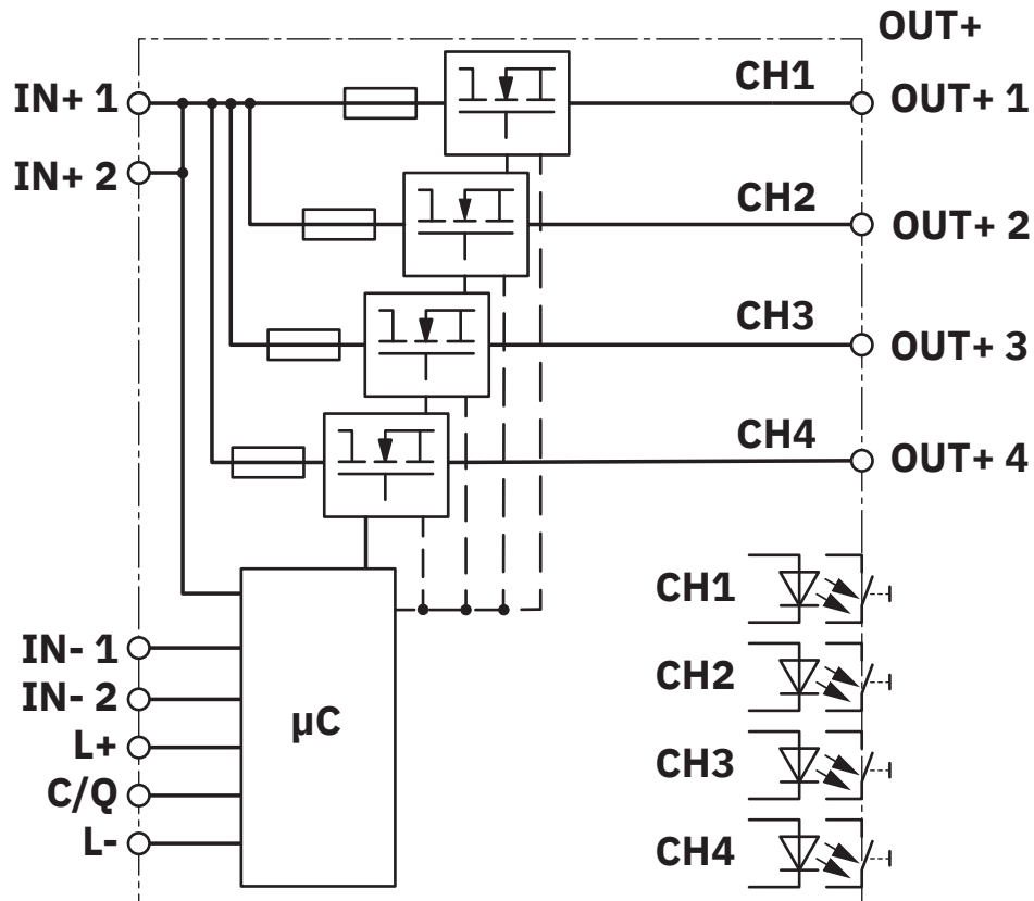
Blokkskjema
