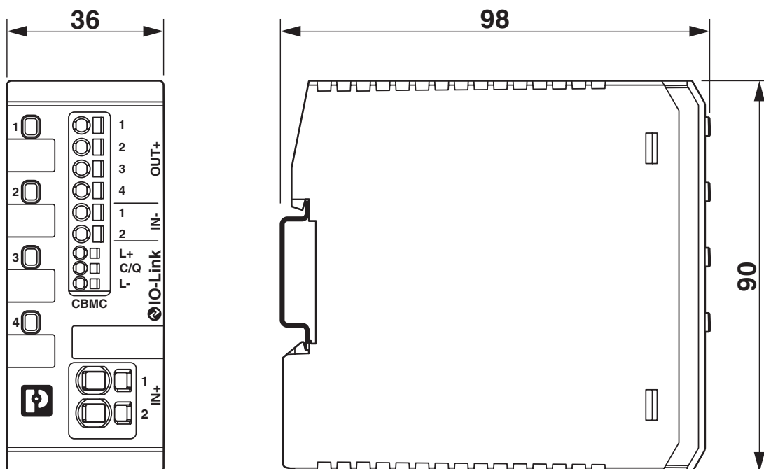
Målskisse
