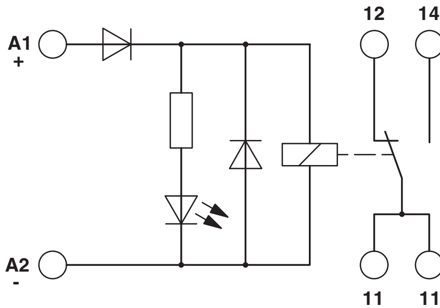
Koblingsskjema
