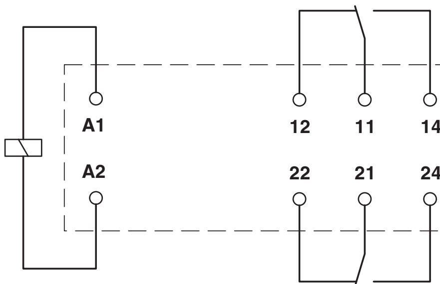
Koblingsskjema
