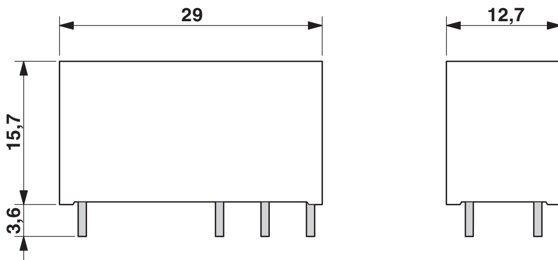
Målskisse
