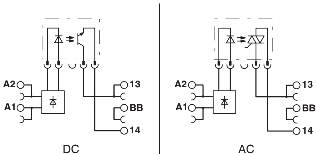
Koblingsskjema
