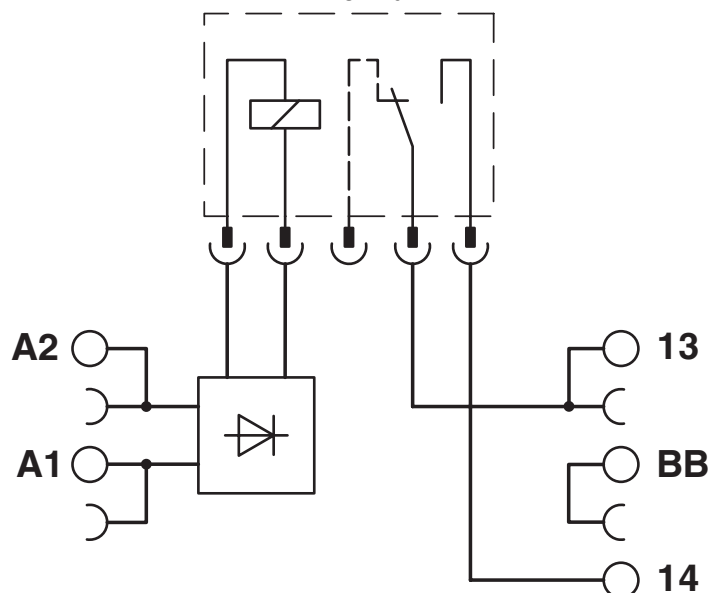
Koblingsskjema
