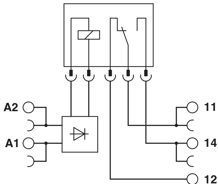
Koblingsskjema
