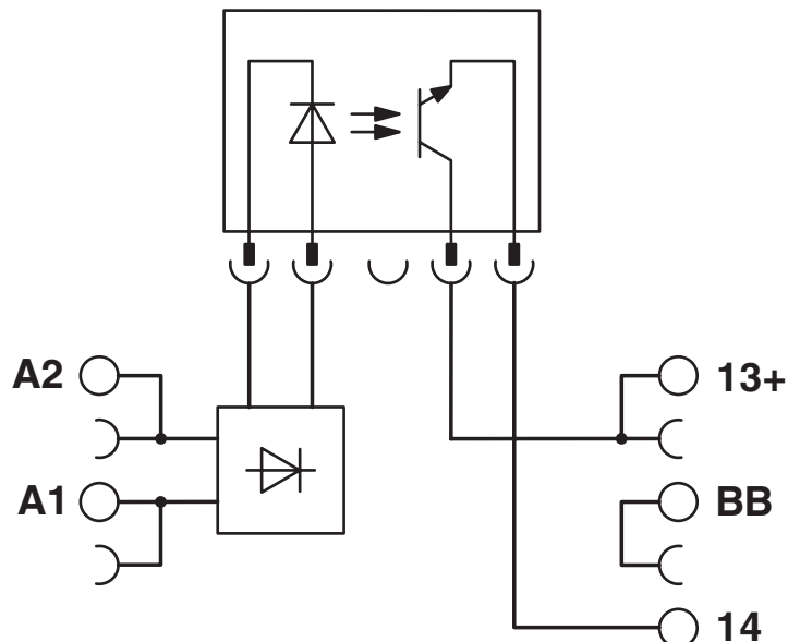
Koblingsskjema
