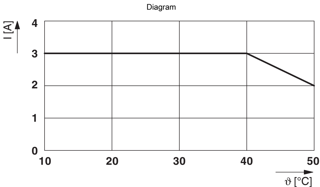
Deratingkurve for varig grensestrøm
