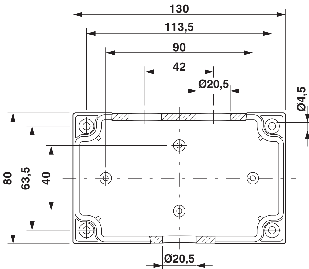
Målskisse
