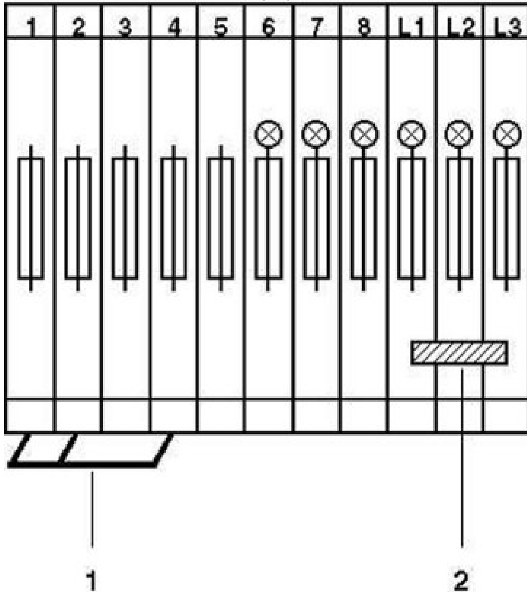
Koblingsskjema
