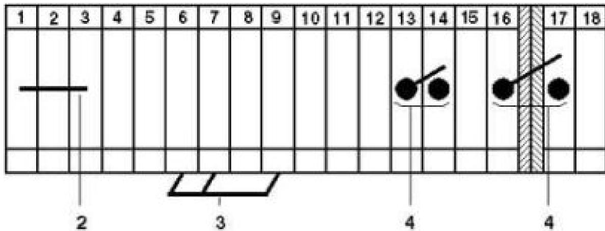
Koblingsskjema
