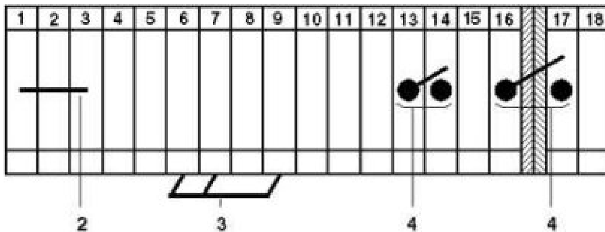
Koblingsskjema
