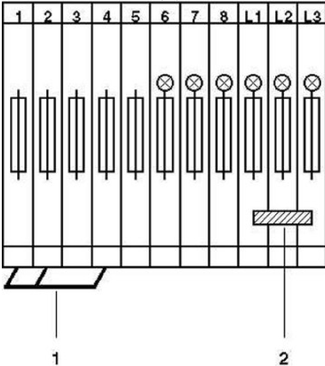
Koblingsskjema
