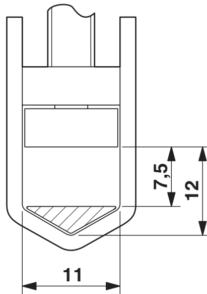
Målskisse
