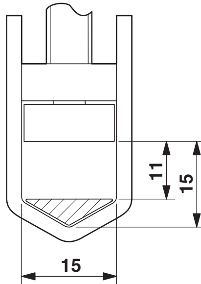
Målskisse
