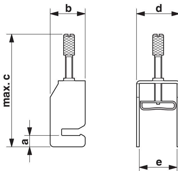
Målskisse
