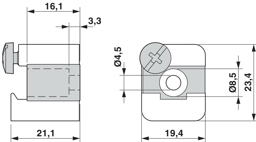
Målskisse
